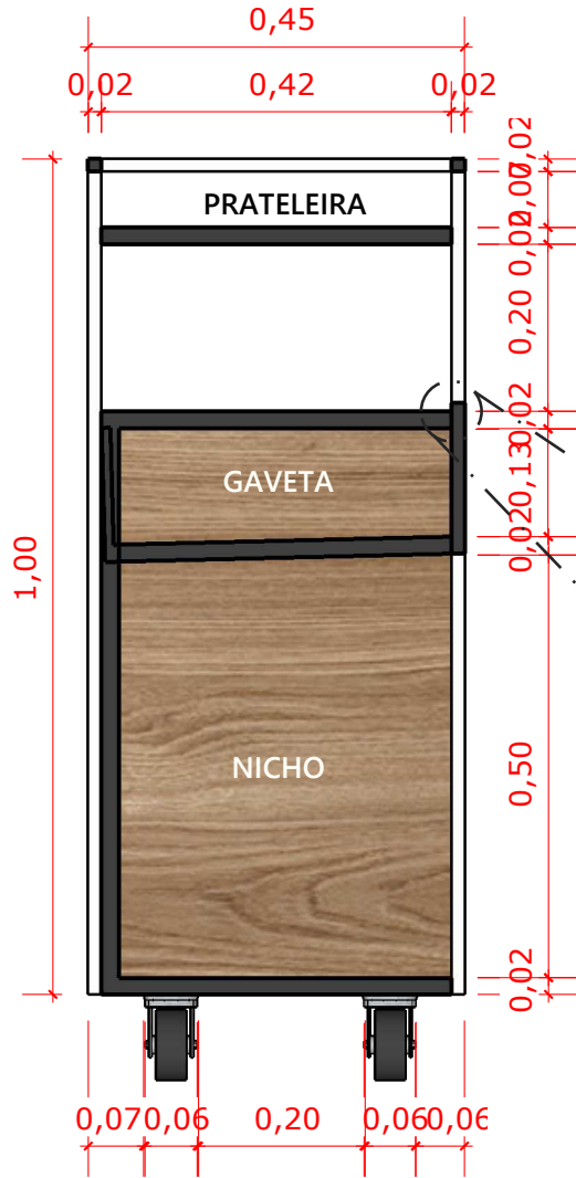
CORTE ESCALA 1/10
