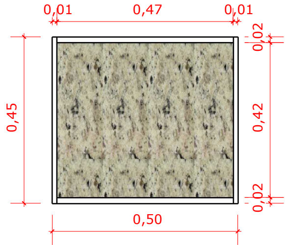
VISTA SUPERIOR ESCALA 1/10
