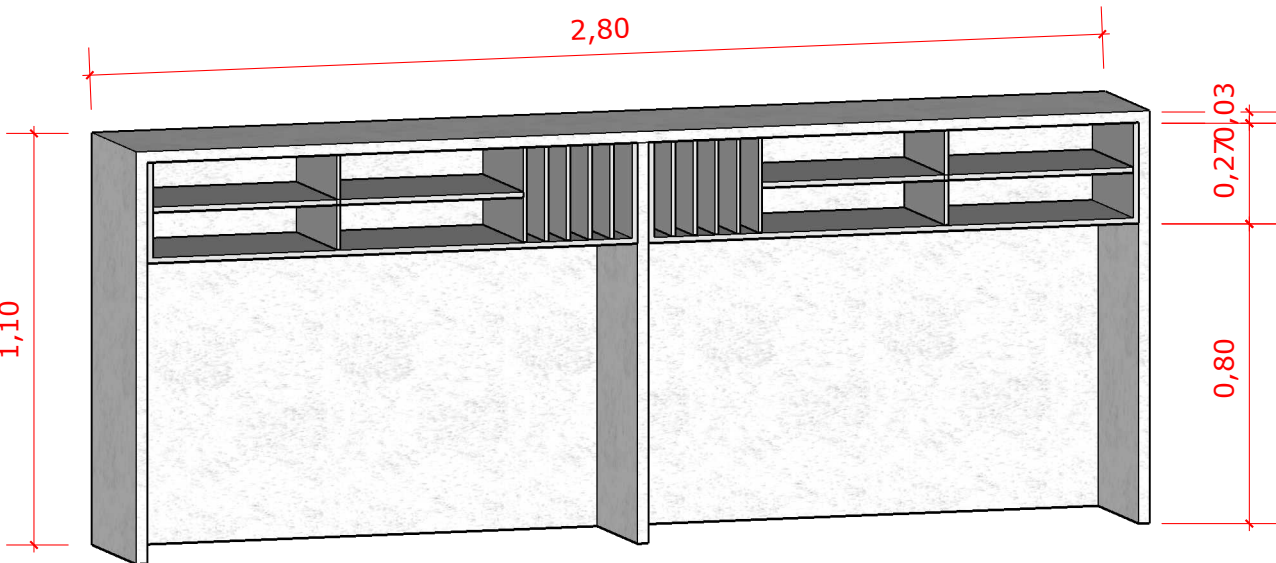
PERSPECTIVA
