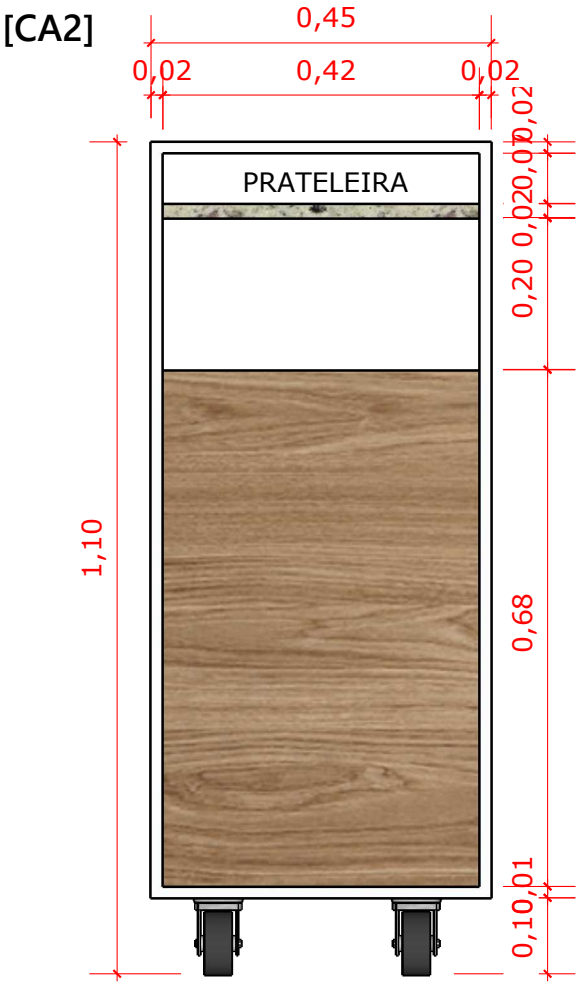
VISTA LATERAL ESCALA 1/10
