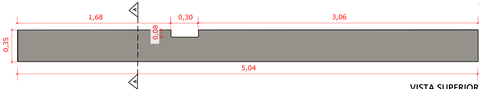
VISTA SUPERIOR ESCALA 1/20
