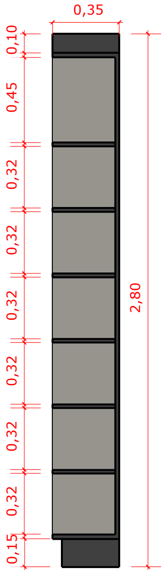
CORTE TRANSVERSAL A ESCALA 1/20
