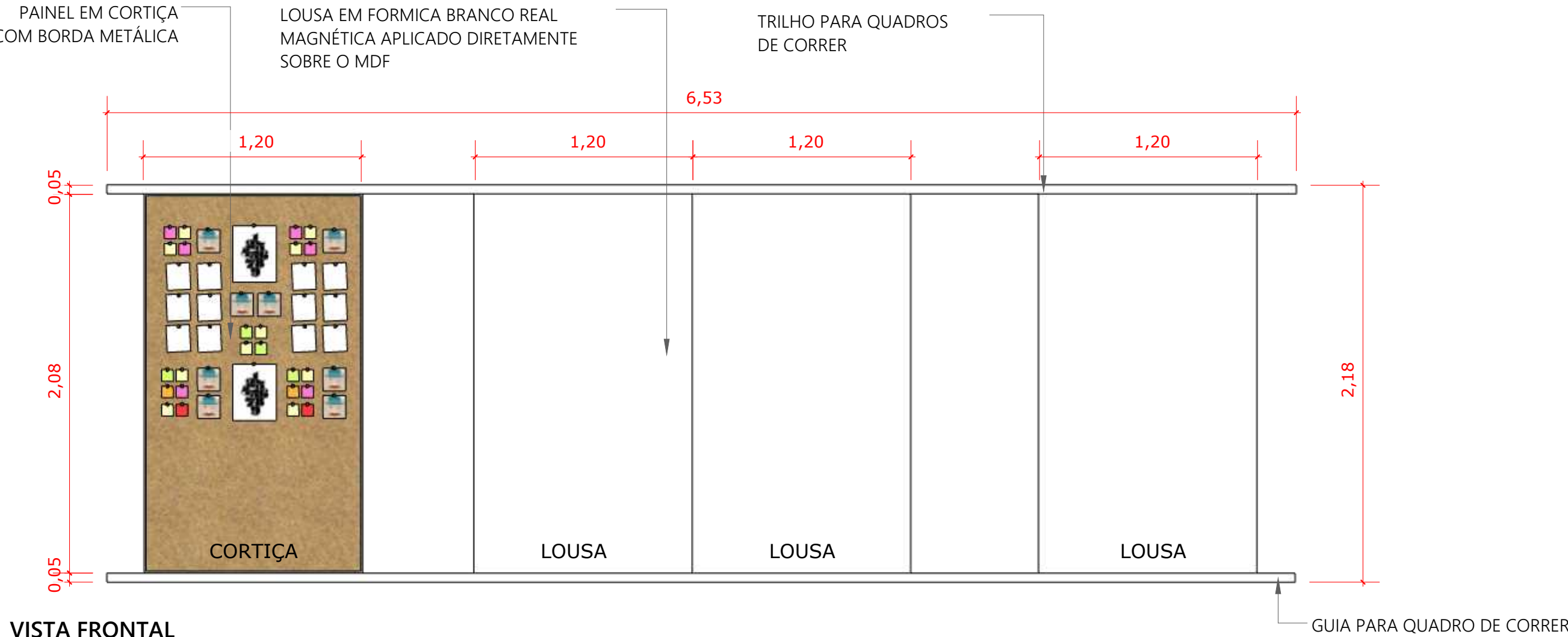
VISTA FRONTAL ESCALA 1/20
