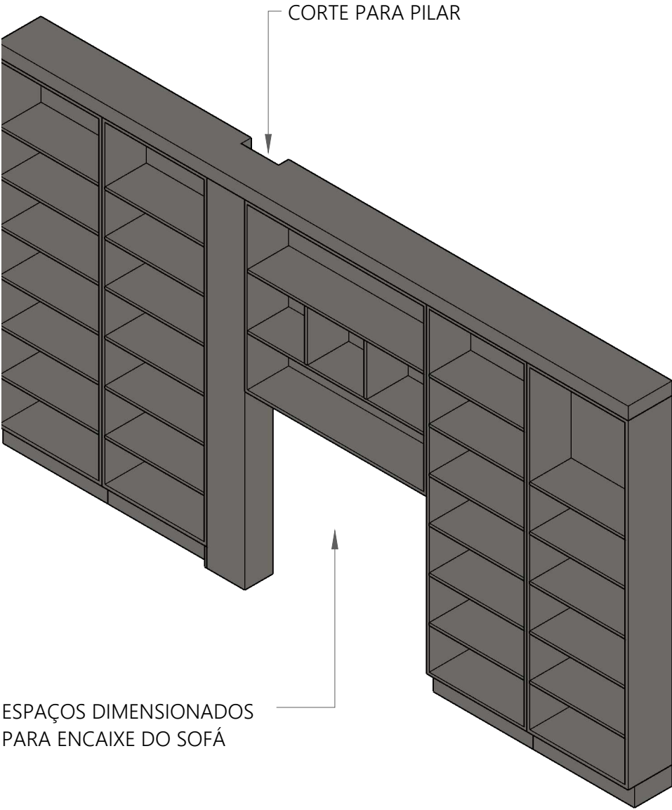
PERSPECTIVA ISOMÉTRICA ESCALA 1/20 (SEM NICHOS)
