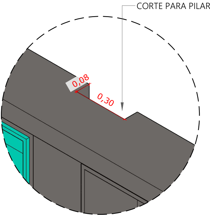
DETALHE 1 ESCALA 1/10
