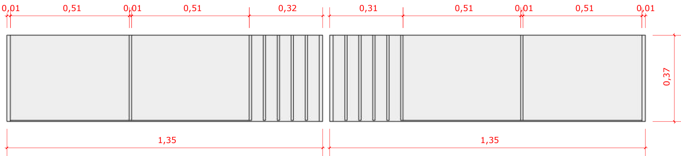
VISTA SUPERIOR
